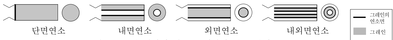
<그림 1> 단면 형상에 따른 그레인의 연소 방식
